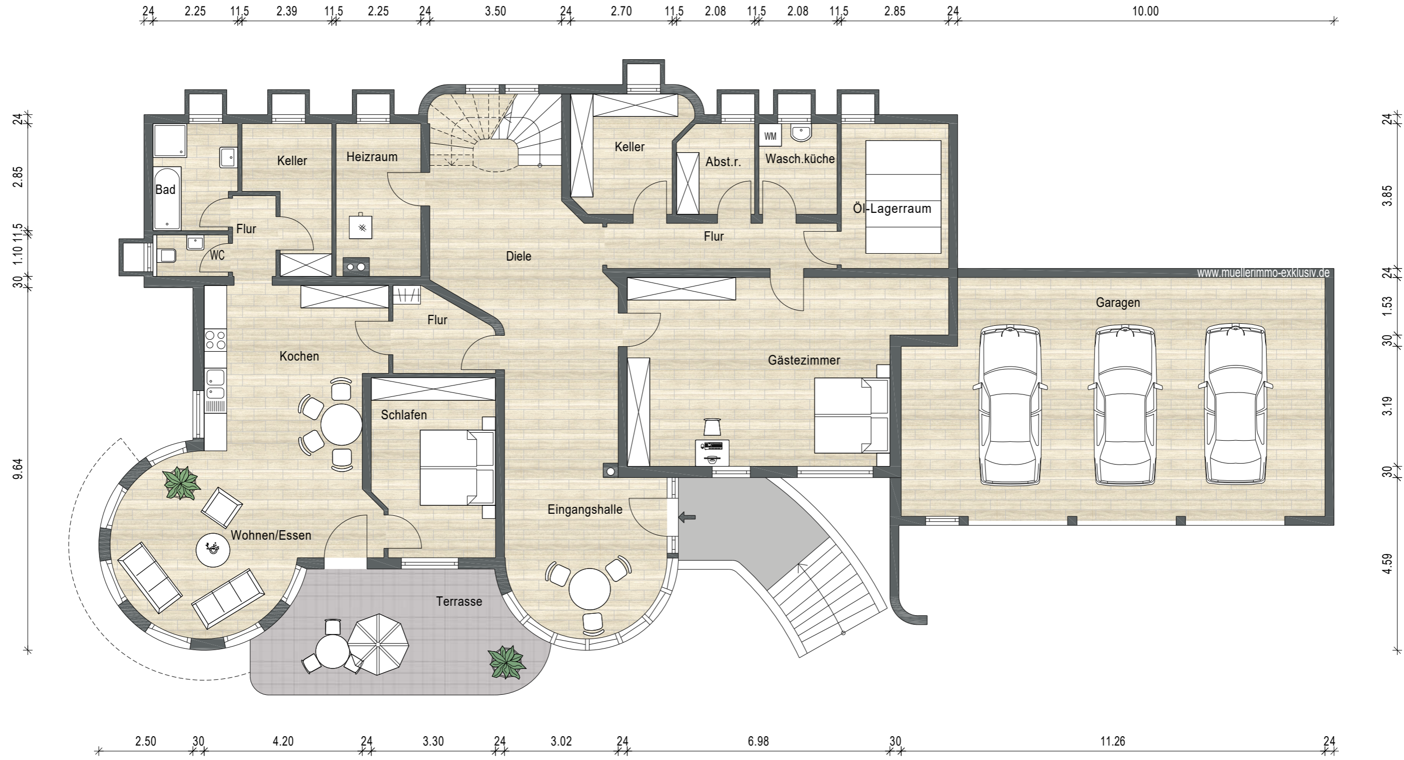
Untergeschoss
